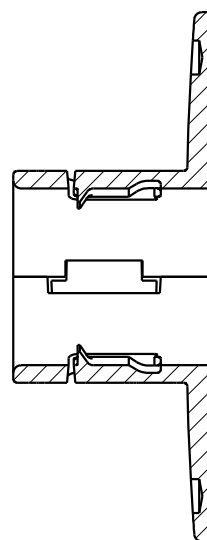
断面 A-A
